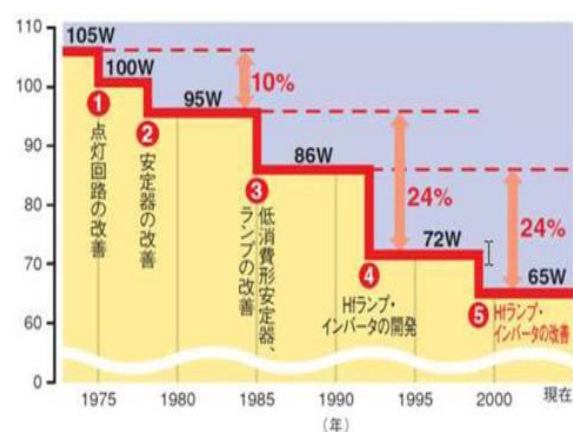
照明器具の消費電力推移
