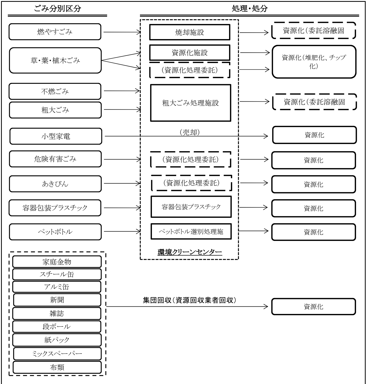
図-1 ごみ処理フロー
