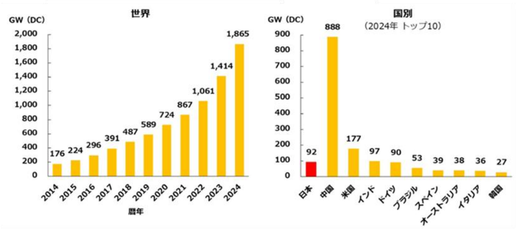
図-1-1 世界の太陽光発電設備容量と国別比較
