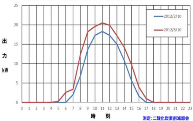
図-1-7 運子市役所 太陽光発電設備 定格 30kW
