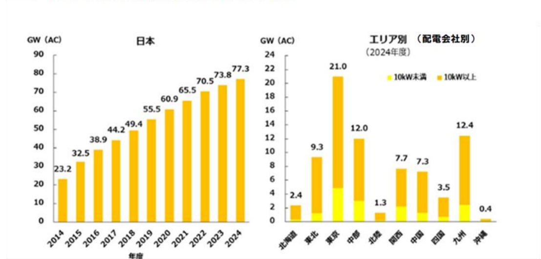
図-1-2 日本の太陽光発電設備容量とエリア別比較
