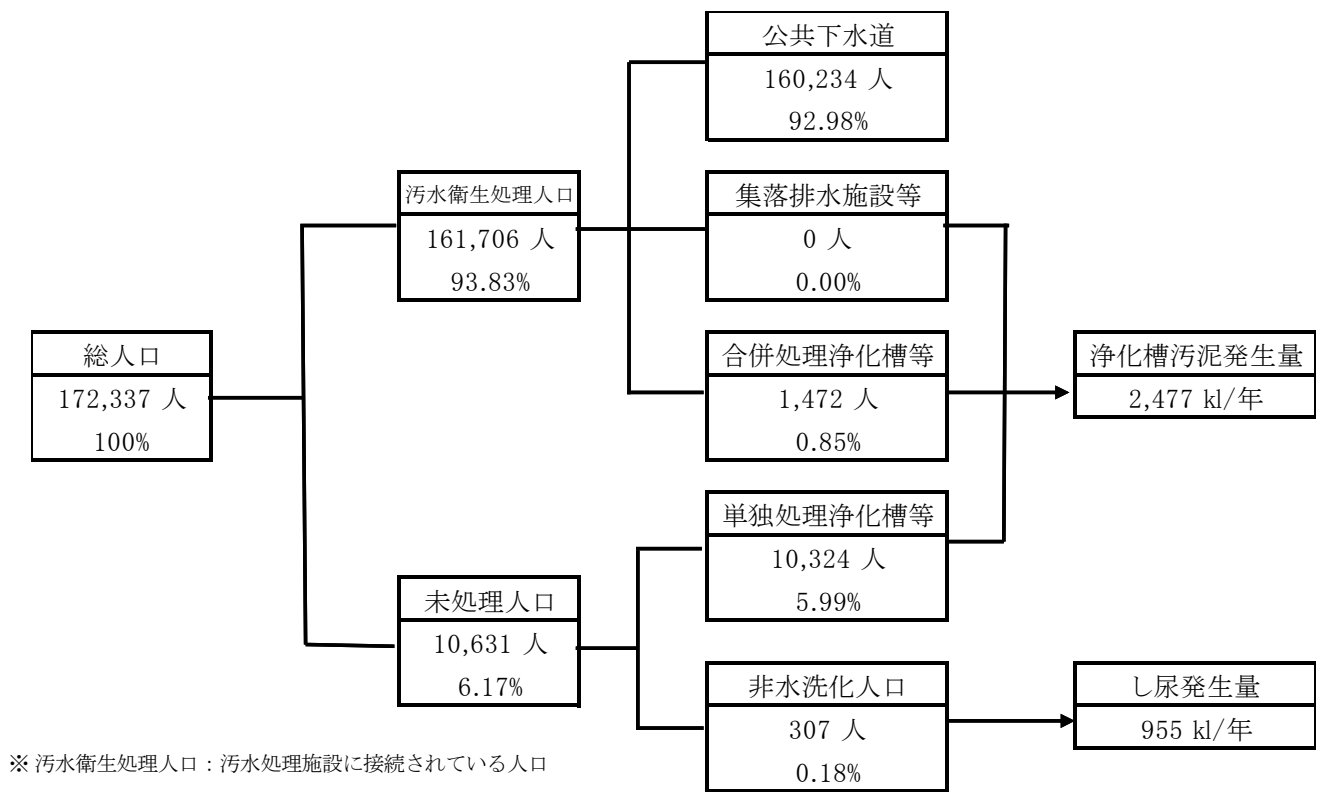
図 3－1 生活排水の処理状況フロー(鎌倉市)
