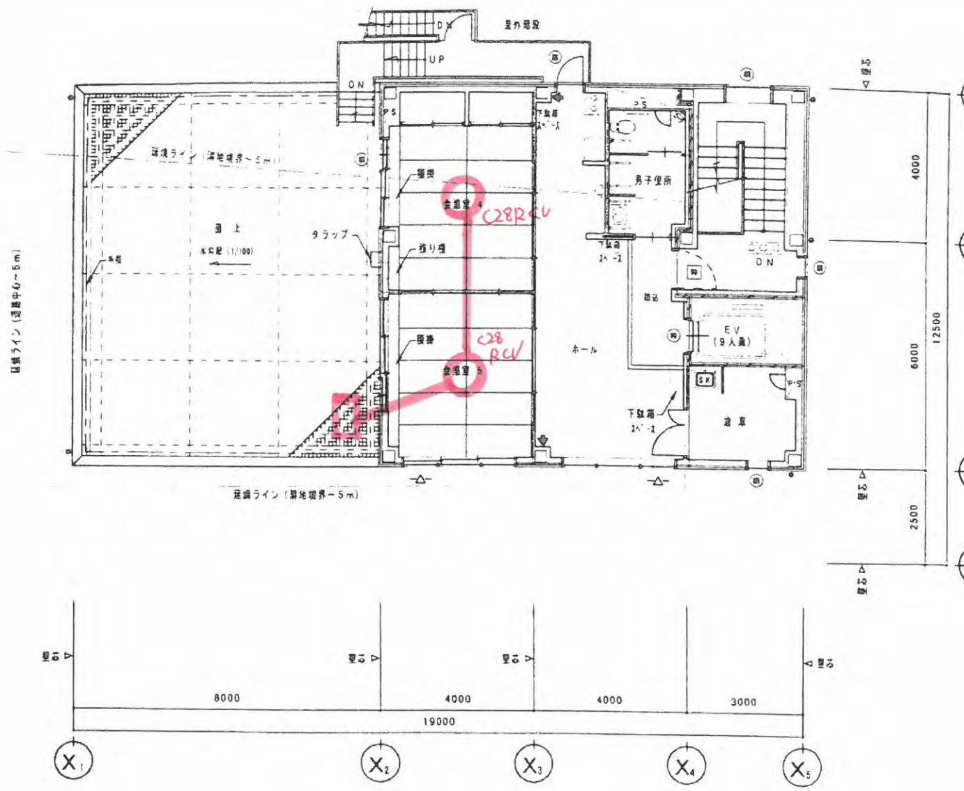
3階平面図
