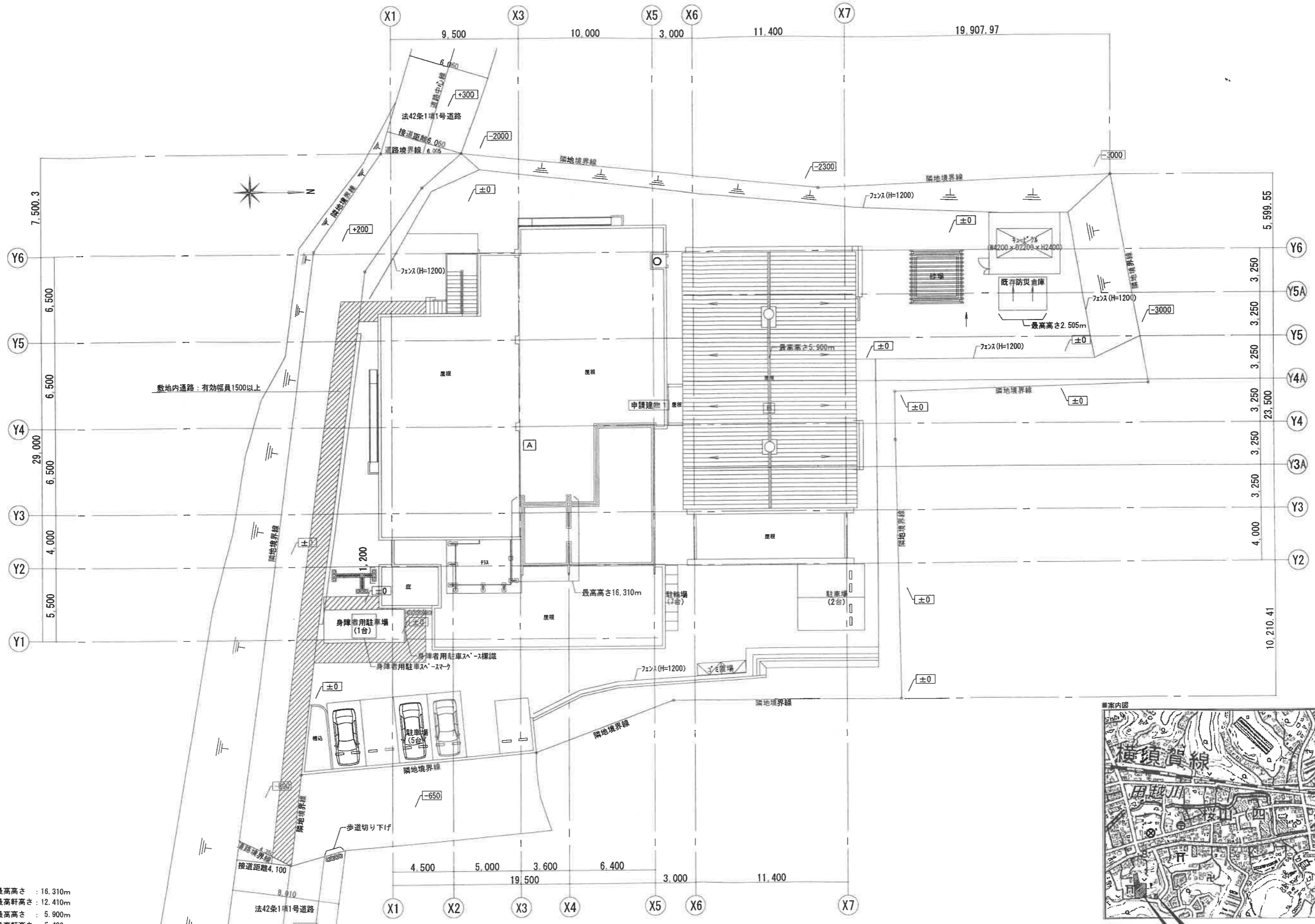
改修配置図
