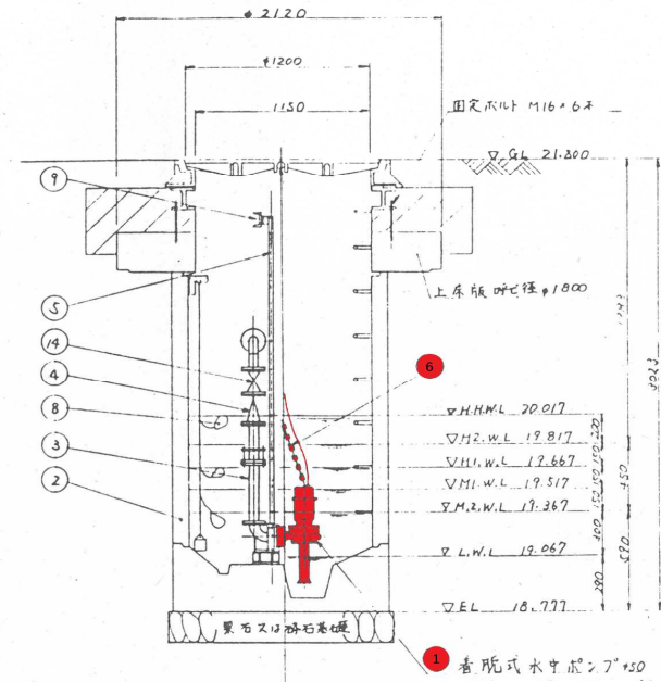
B-B断面
