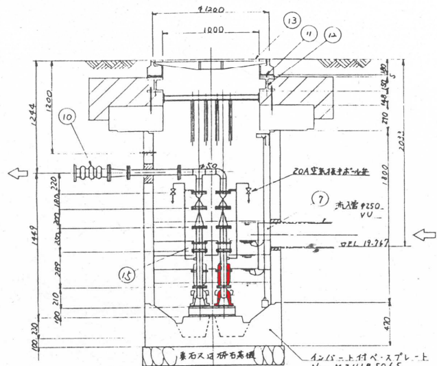
A-A断面
