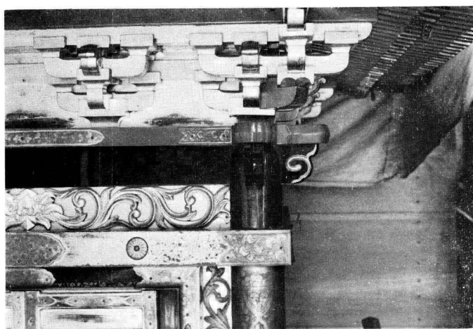
池子神明社 神輿軒斗拱
