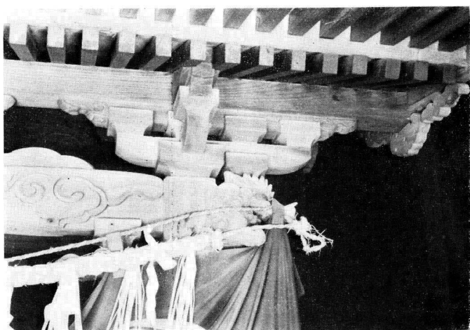
伊勢町八幡宮 本殿向拝細部
