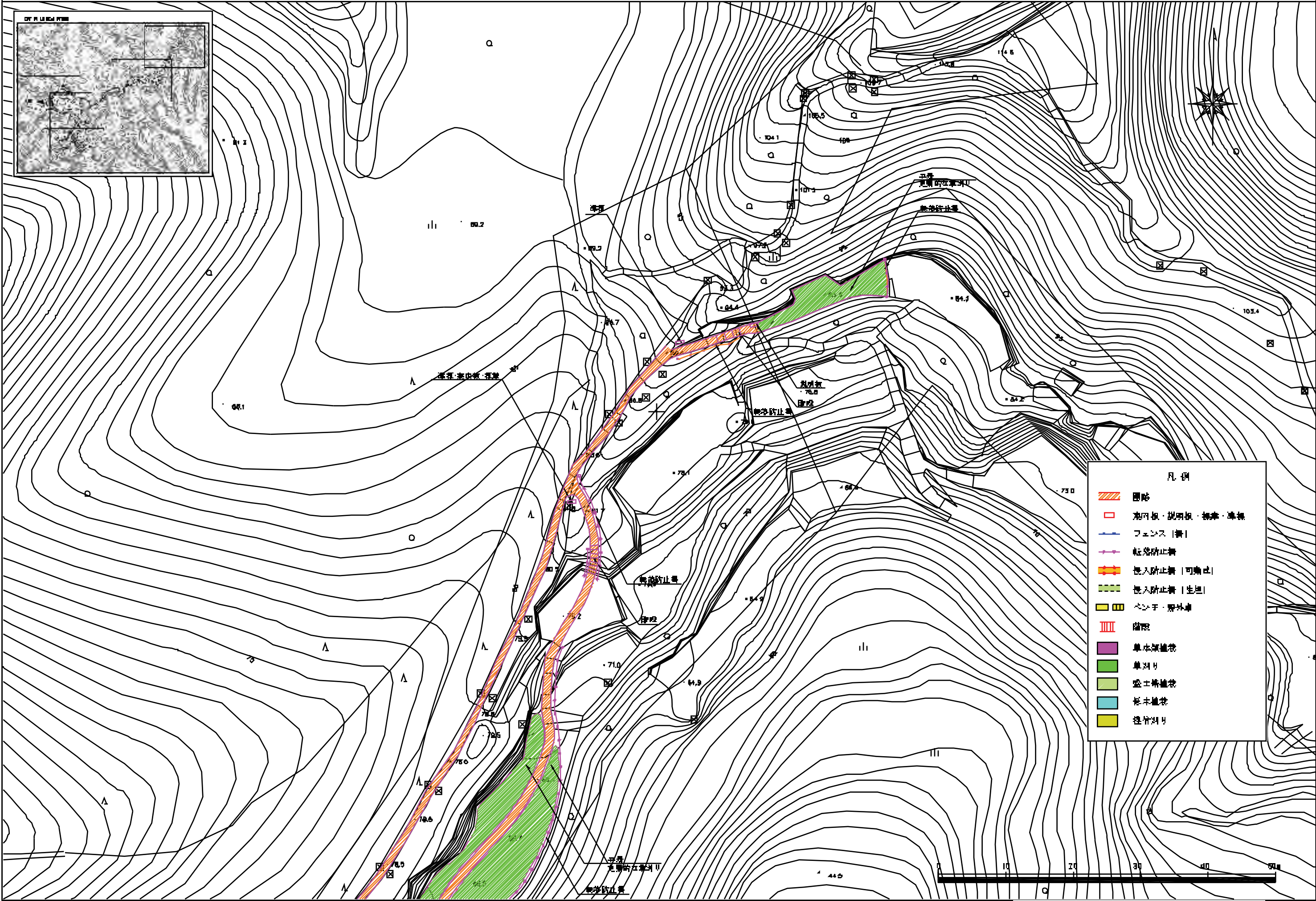
図4-23 大切岸・石切跡エリア拡大計画平面図
