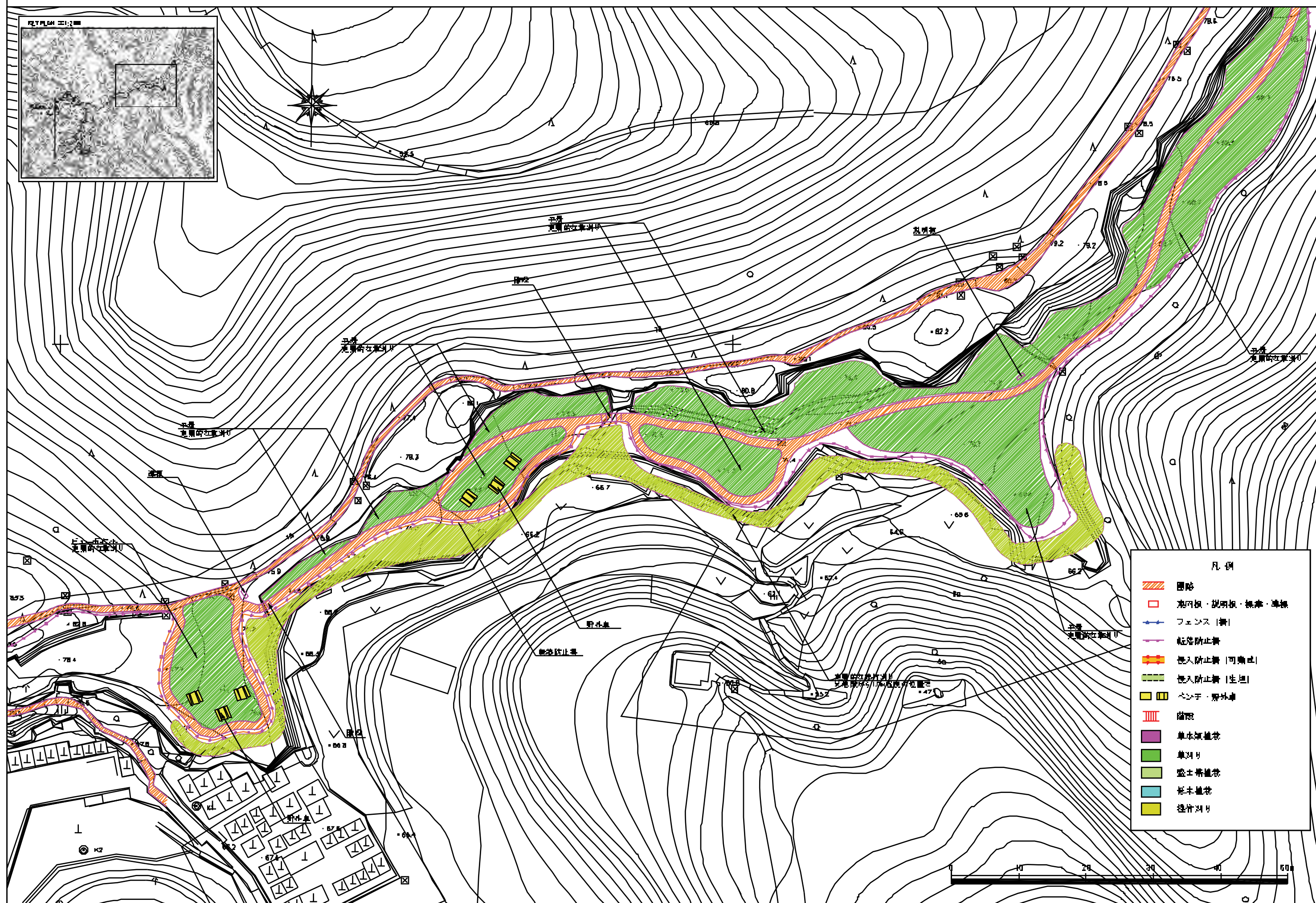
圖4-22 大切岸エリア拡大計画平面図
