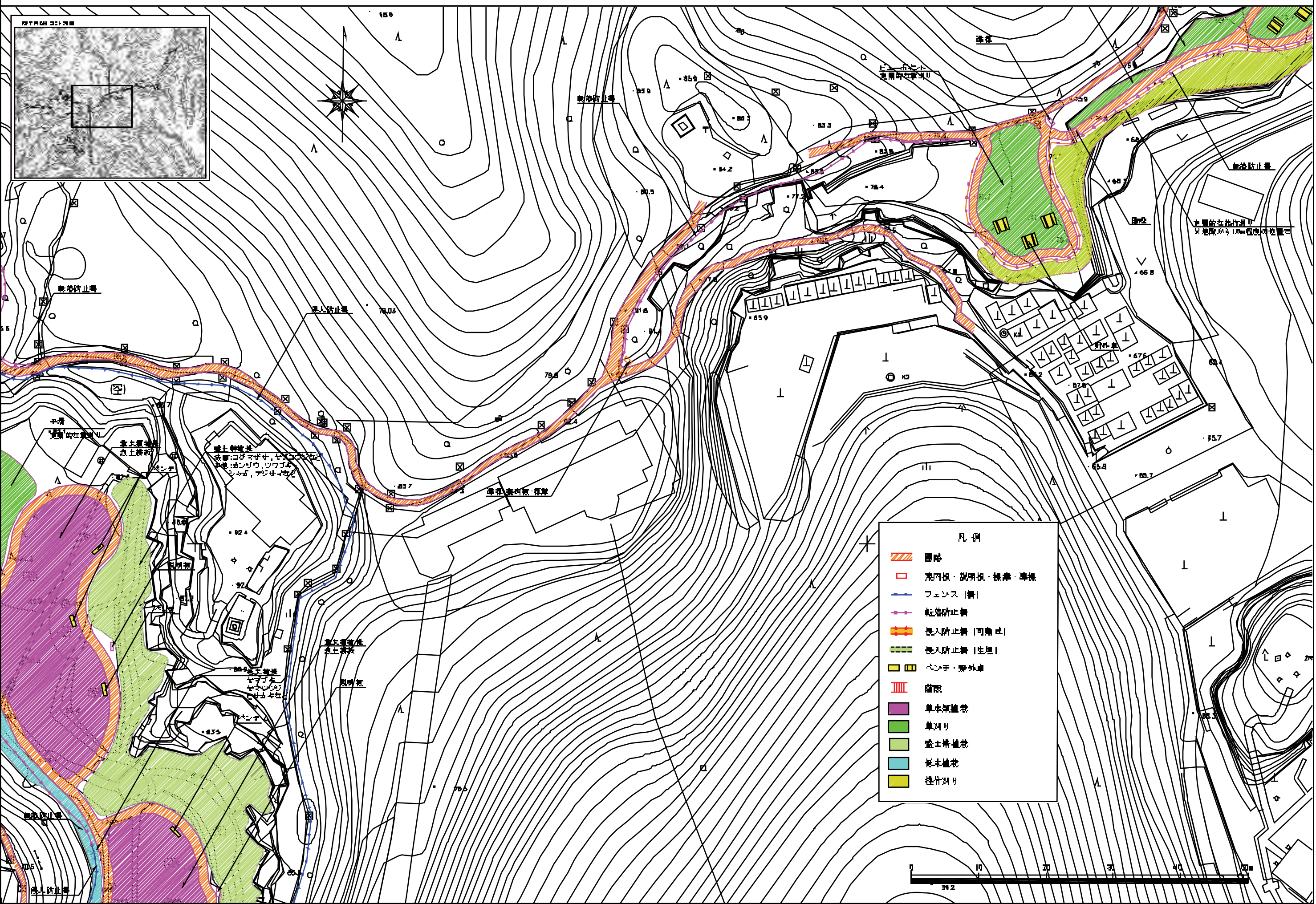
図4-21 まんだら堂やぐら群東側エリア拡大計画平面図
