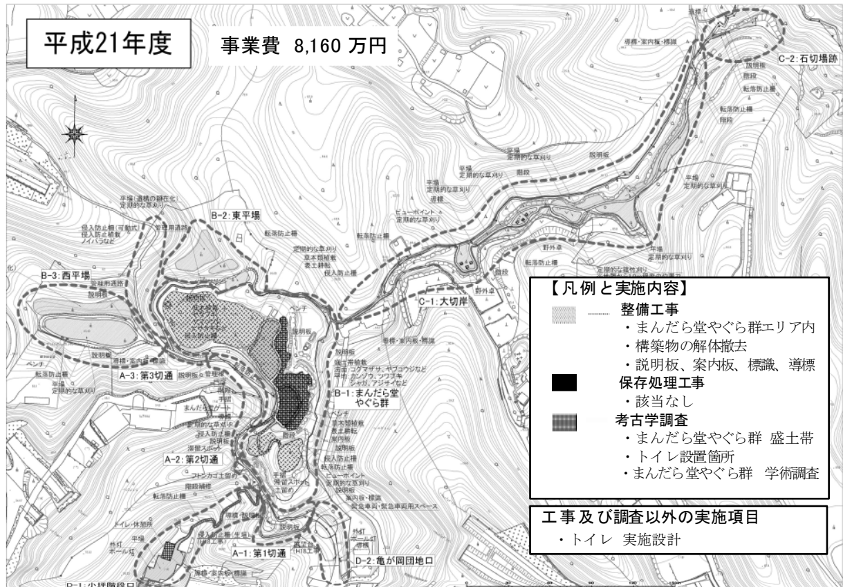
図7-3 年度別整備計画平面図（短期整備・平成21年度）
