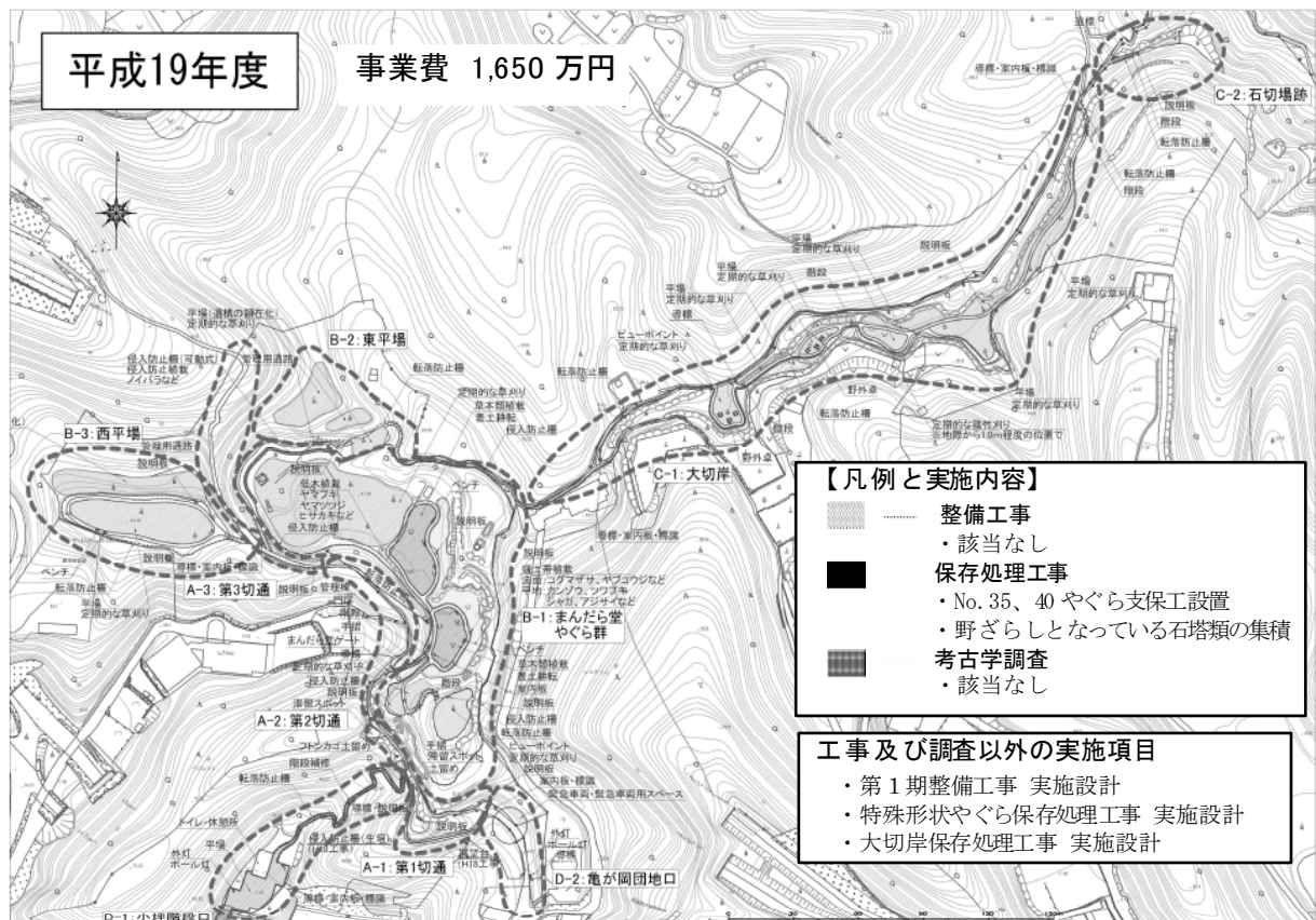
図7-1 年度別整備計画平面図（短期整備・平成19年度）
