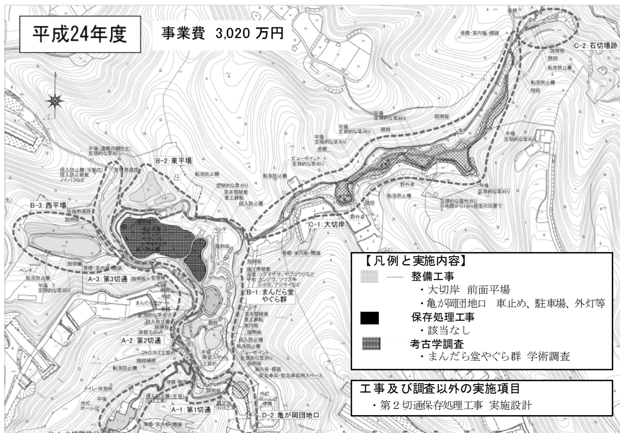
図7-6 年度別整備計画平面図（中期整備・平成24年度）
