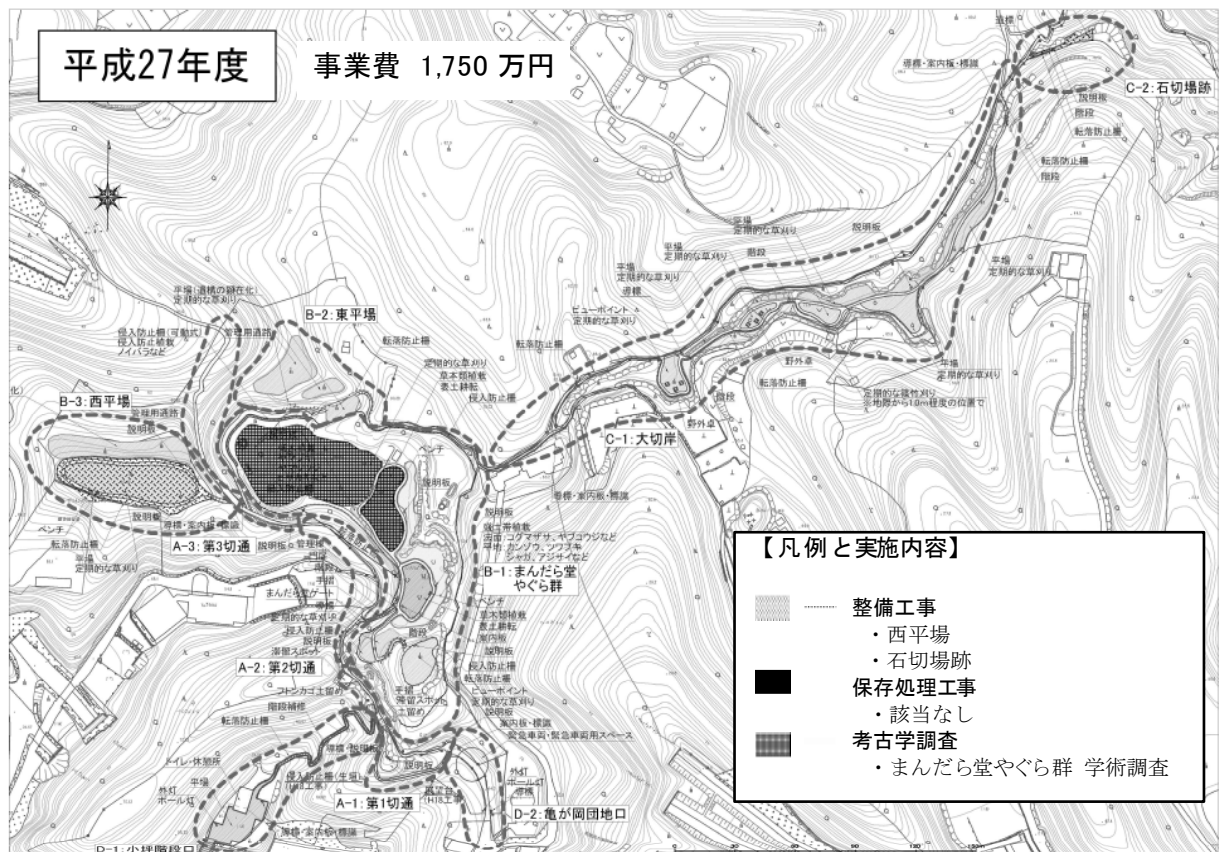
図7-9 年度別整備計画平面図（長期整備・平成27年度）
