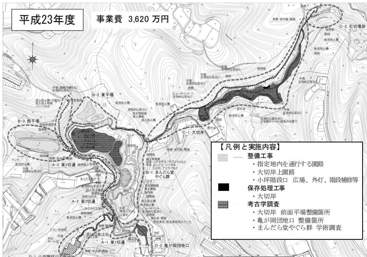
図7-5 年度別整備計画平面図（中期整備・平成23年度）
