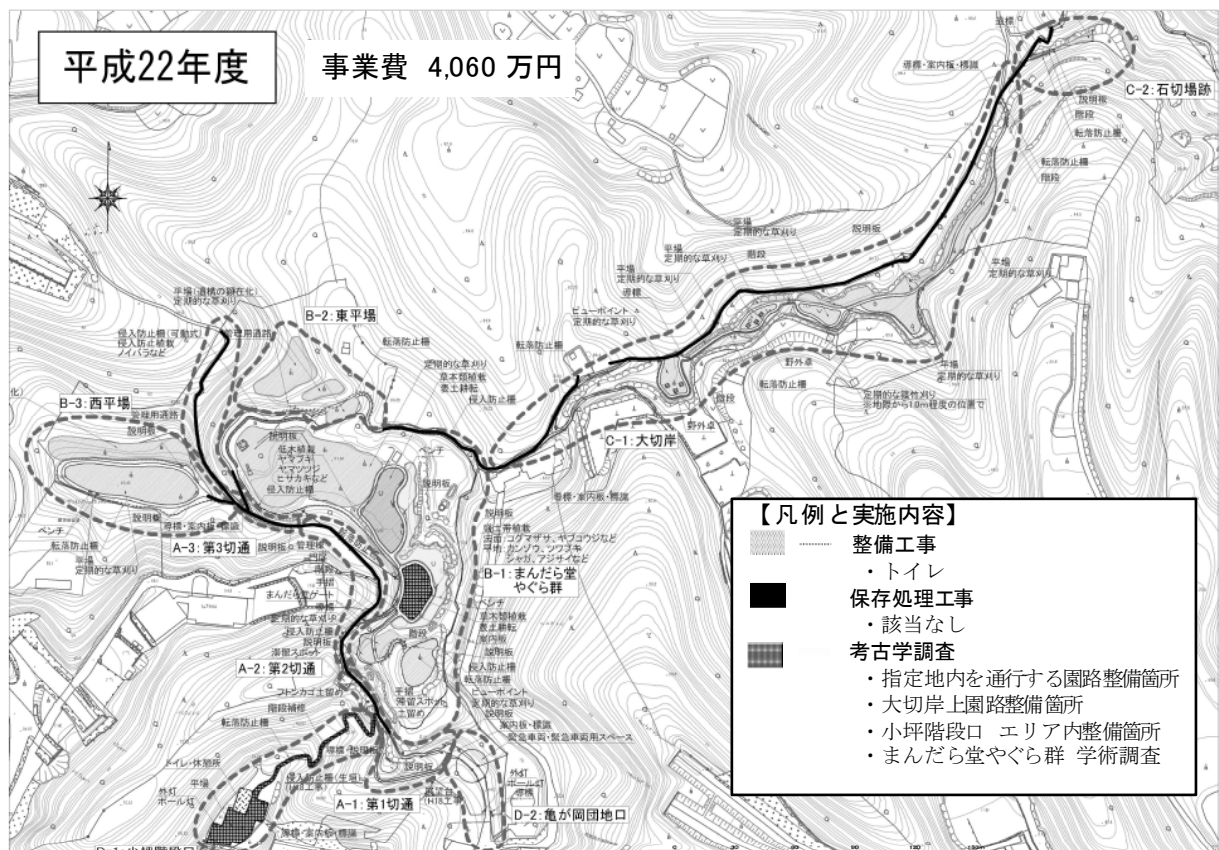
図7-4 年度別整備計画平面図（中期整備・平成22年度）
