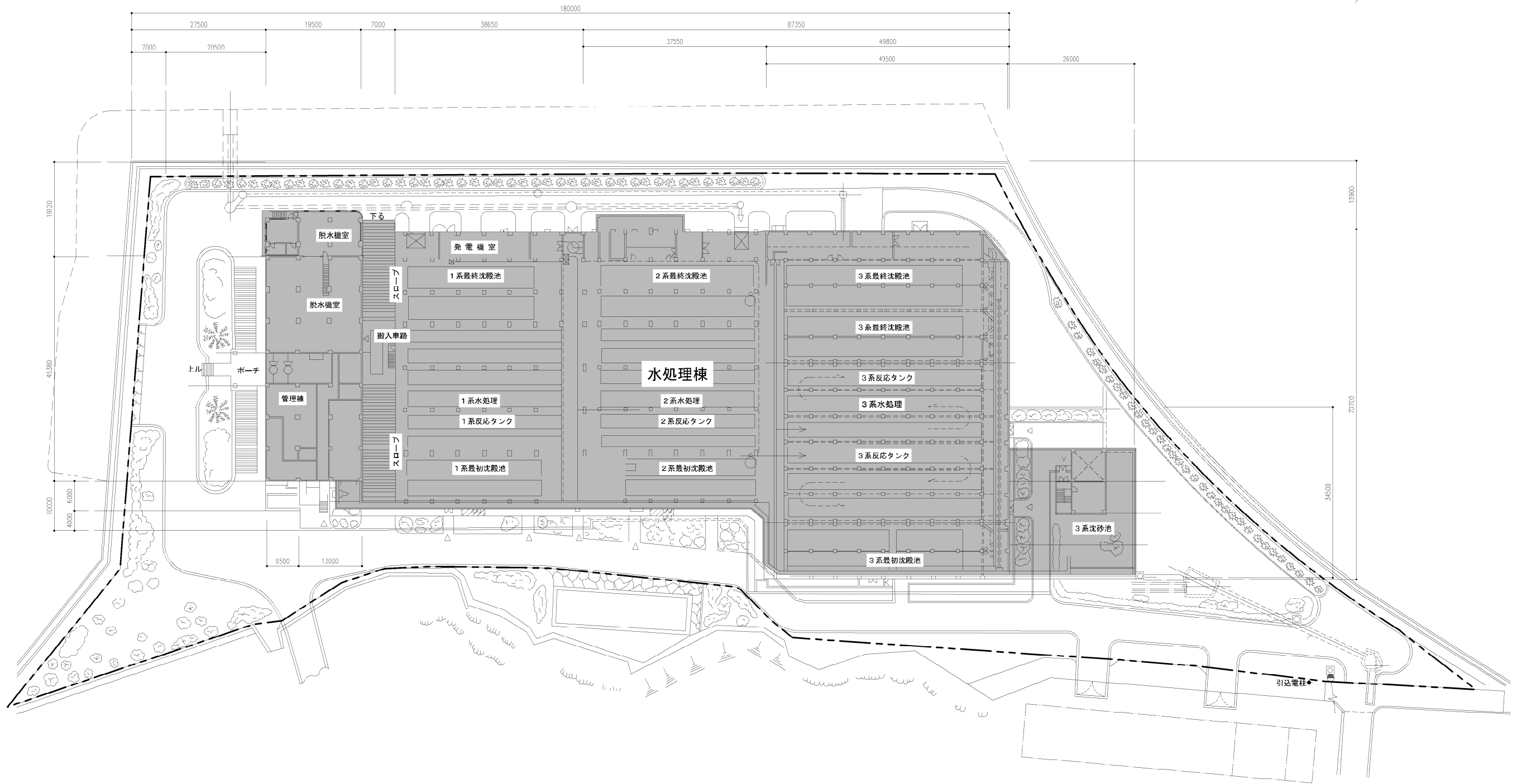
全体配置図 s=1/400
